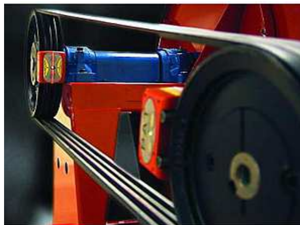
Thiết bị căn chỉnh đồng tâm Puly bằng laser Laser pulley alignment tool
