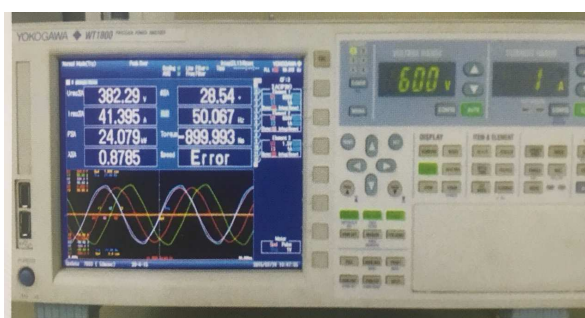
Thiết bị đo tổng hợp công suất WT1800 Power analyzer WT 1800
